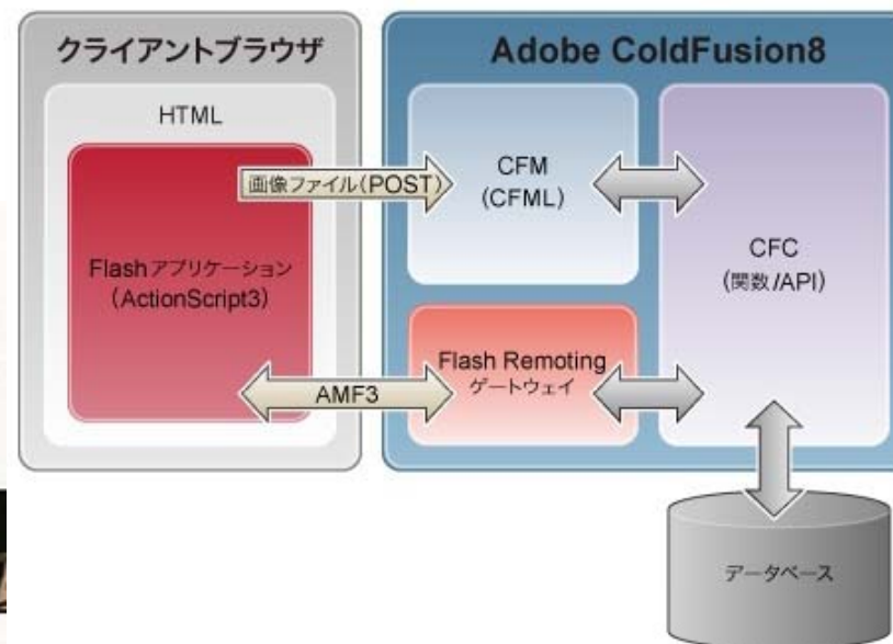
フロントエンドのアプリケーション構成図
